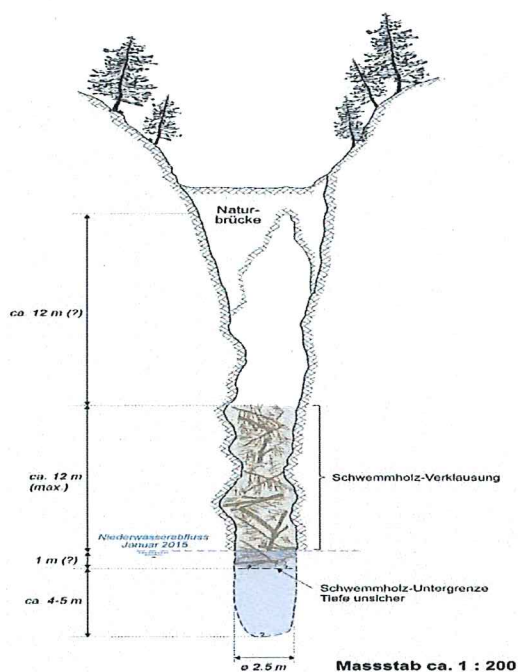
Skizze der Schwemmholz-Verkläusung beim Räbloch (Quelle: Geotest AG, 2015)
